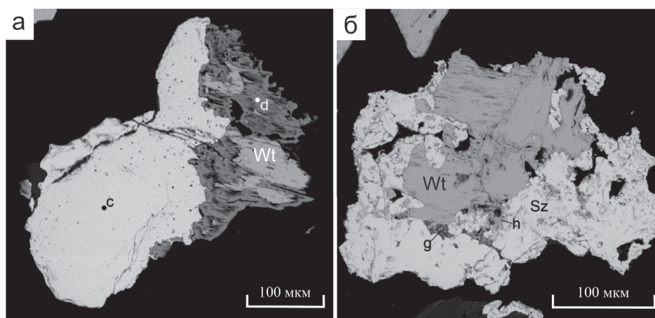
Рис. 12. Вторичные минералы вольфрама: а – сросток штольцита (точка с, ан. 2 в табл. 5) и оксигидроксидов Mn (d), замещающих гюбнерит (Wt); б – сросток урансодержащих фаз (точка g, ан. 4, точка h, ан. 5 в табл. 5) с гюбнеритом (Wt) и штольцитом (Sz).
