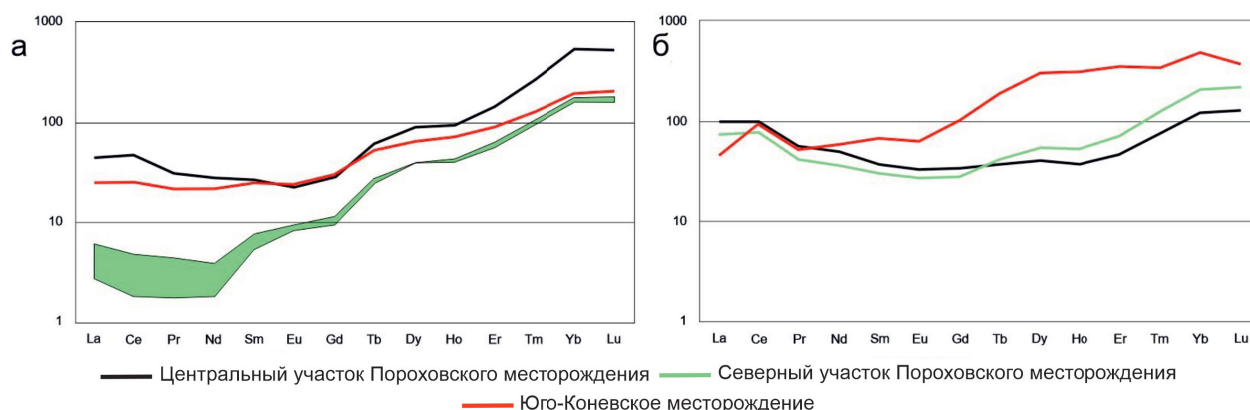
Рис. 8. Распределение РЗЭ в вольфрамите первичных (а) и окисленных (б) руд. Fig. 8. REE pattern of wolframite from primary (a) and oxidized (б) ores.
