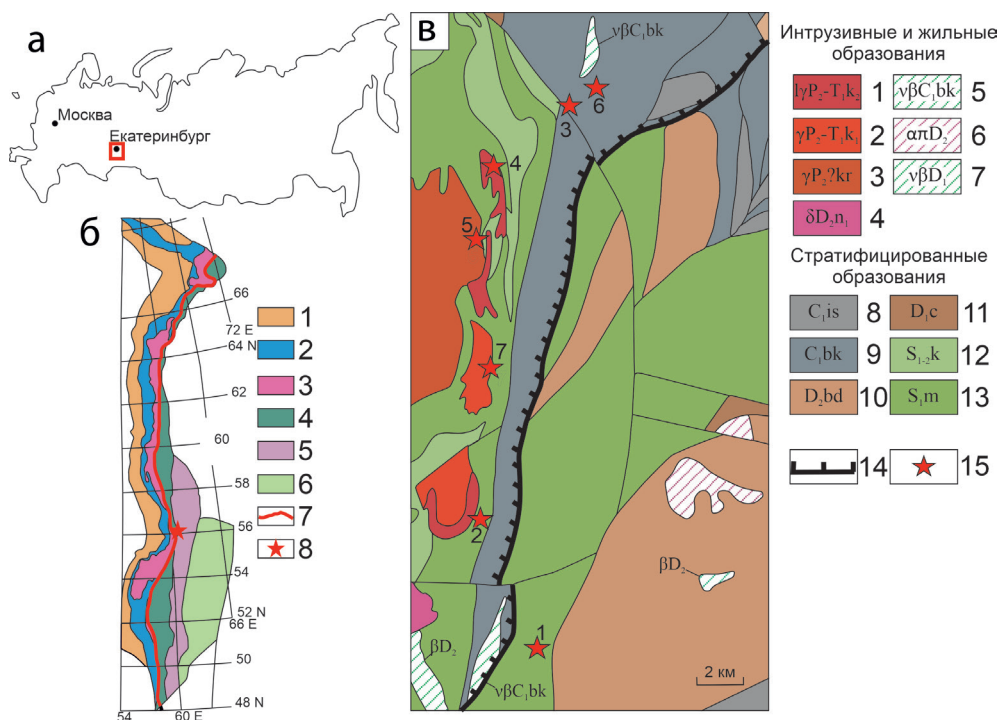
Рис. 1. Положение месторождений Коневско-Карасьевского рудного узла на географической схеме (а), схеме тектоно-магматического районирования Урала (Puchkov, 2017) (б) и схеме рудного узла (Коровко и др., 2015) (в).
