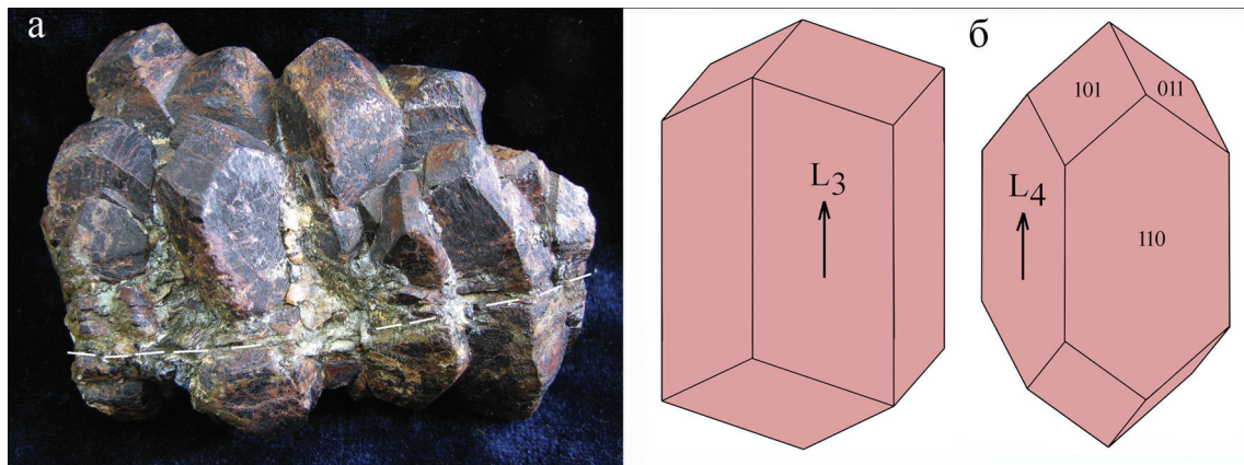
Рис. 4. Асимметрия ромбододекаэдров метакристаллов альмандин: а – друза кристаллов, выросших от трещины во вмещающие хлоритовые сланцы; б – модели ромбододекаэдров, удлинённых вдоль тройной ( L_3 ) и четверной ( L_4 ) осей. Размер образца 4 см.
