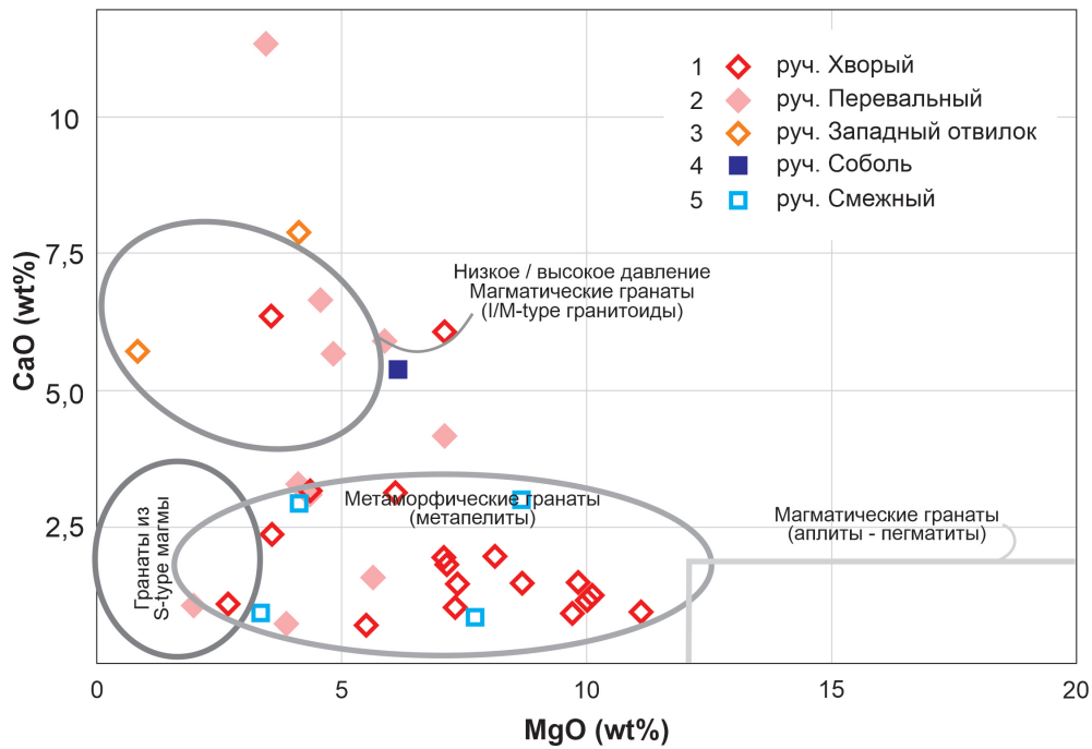
Рис. 8. Соотношение содержаний MnO и CaO в гранатах из шлиховых проб, отобранных из водотоков бассейна руч. Анмандыкан 2-ой.
