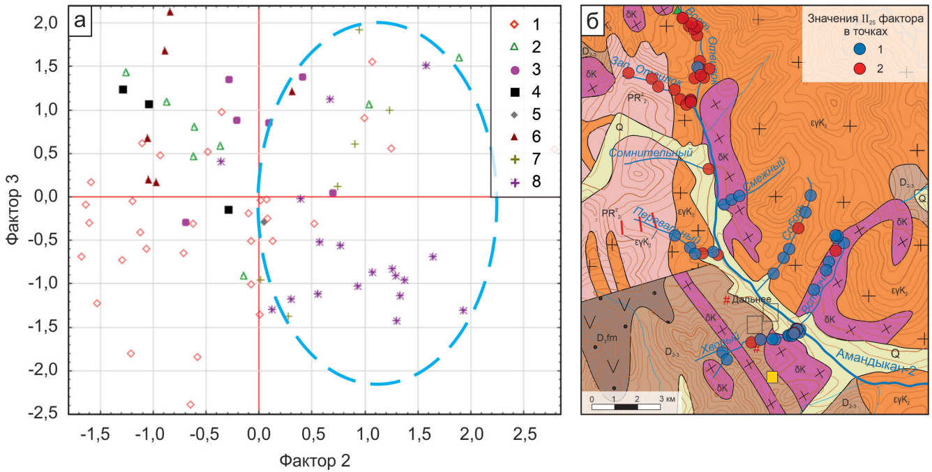
Рис. 10. а – диаграмма значений факторов II и III: голубая линия – положительные нагрузки фактора II (Pb); б – картосхема значений фактора II в точках отбора шлиховых проб. Fig. 10. а – diagram of values of factors II and III in the points: blue line – positive values of factor II (Pb); б – schematic map of values of factor II in sampling points.
