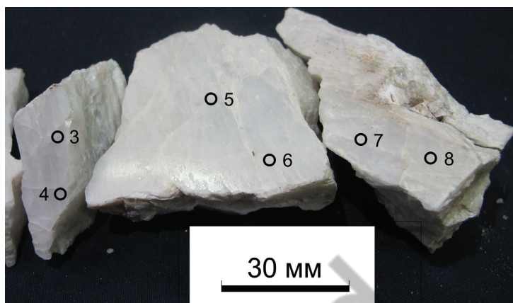
Рис. 5. Обломки кристалла сподумена из пегматита блоковой структуры с указанием точек анализа (обр. № 3).
