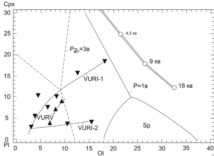
Рис. 9. Положение средних нормативных составов магматитов верхнеуральской ассоциации на диаграмме плаво-к-сти системы «плаггиоклаз–клинопироксен–оливин» (Фролова и др., 1989).
