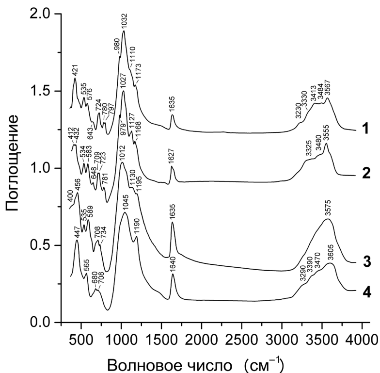
Рис. 5. Инфракрасные спектры цеолитов: 1, 2 – гускрикит из Булатовского карьера (1) и карьера близ г. Насик, Махараштра, Индия (2); 3 – брюстерит-Sr с эмпирической формулой (Sr 1.4 Ba 0.6 K 0.1 )(Si 11.9 Al 4.1 O 32 ) · nH 2 O из рудника Уайтсмит, Стронтиан, Шотландия; 4 – эпистильбит из карьера Шиаторска Буковинка, Банска Бистрица, Словакия.
