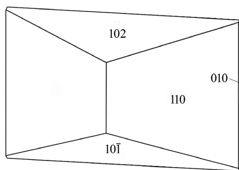
Рис. 4. Чертеж кристалла гускрикита. Fig. 4. Drawing of the gooselickite crystal.
