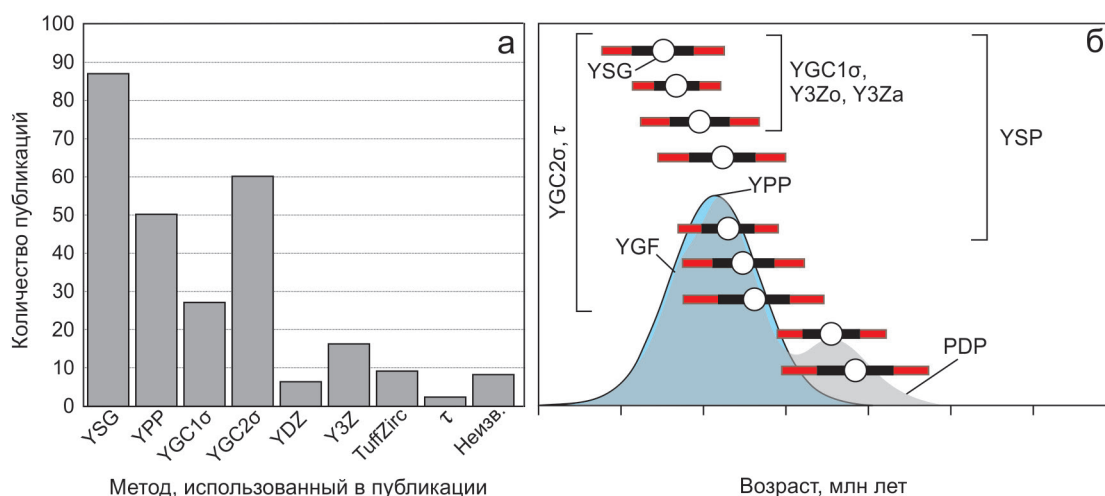
Рис. 8. а – распространение методов MDA, использованных в публикациях, с упрощениями по (Coutts et al., 2019). Методы: YSG – самое молодое зерно; YPP – самый молодой графический пик; YGC 1σ – самый молодой кластер зерен с неопределенностью 1σ; YGC 2σ – самый молодой кластер зерен с неопределенностью 2σ; YDZ – самый молодой детритовый циркон; Y3Z – средневзвешенное трех самых молодых цирконов; TuffZirc – алгоритм TuffZirc; τ – метод τ, взвешенное среднее дат, попадающих в самый молодой пик вероятности; Неизв. – неизвестный алгоритм выбора цирконов; б – различия в методах определения MDA на диаграмме распределения плотности вероятности. YGF – метод самого молодого гауссова пика (Nielsen et al., 2024).
