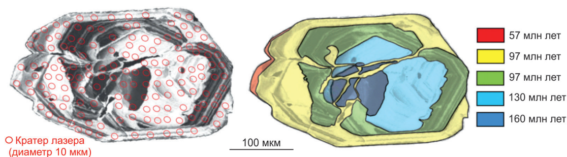
Рис. 3. Катодолюминесцентное изображение циркона со сложной ростовой зональностью, отражающей многократное растворение и регенерацию в течение 100 млн лет (Gehrels, 2012).
