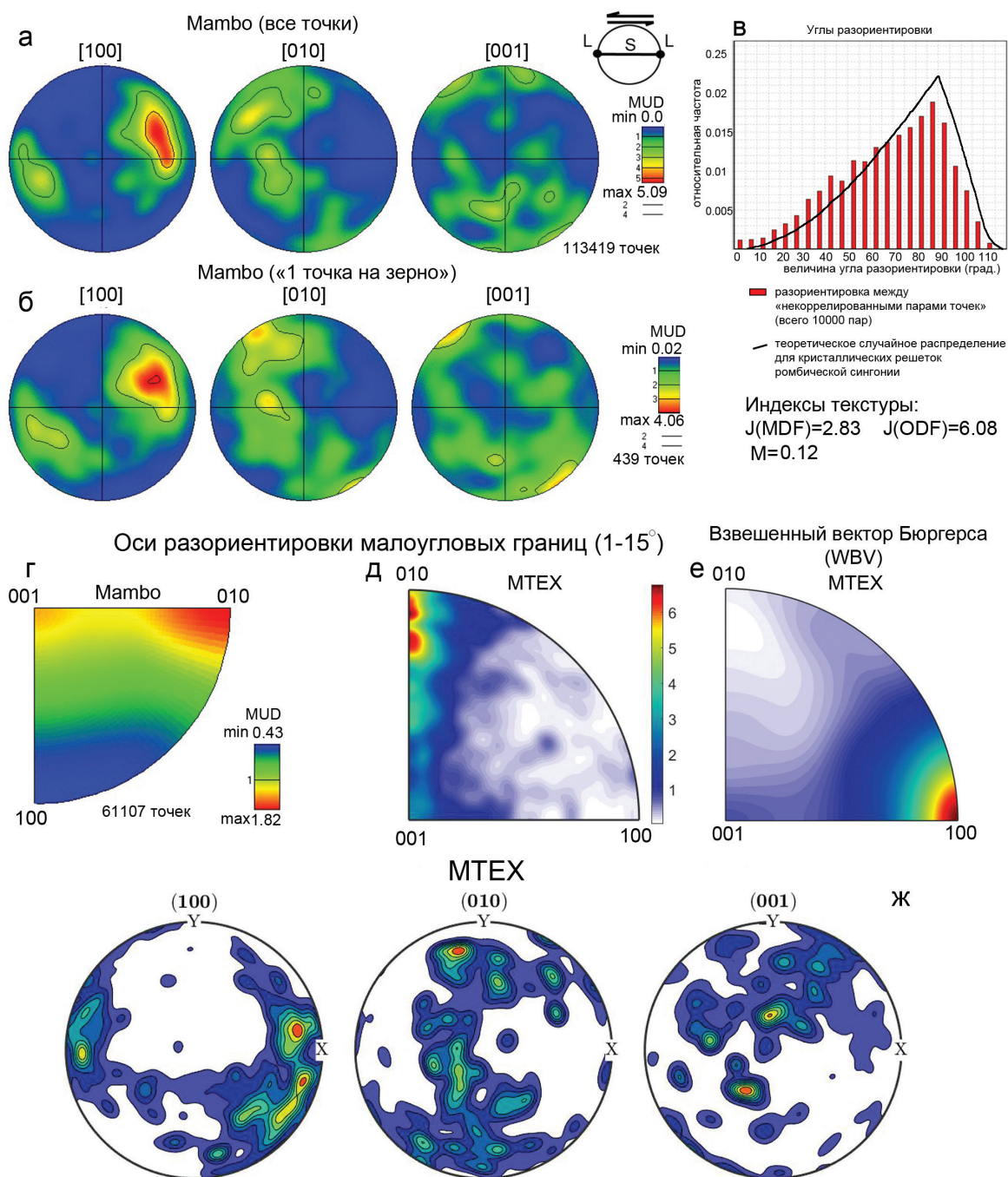
Рис. 4. Текстуальные характеристики образца дунита KN-2020: а, б – прямые полюсные фигуры для оливины, полученные в программе Mambo (равноплощадная проекция на верхнюю полусферу, полуширина 20°): а – обработаны все точки; б – режим «1 точка на зерно»; в – гистограмма распределения углов разориентировки для пар некоррелированных (случайно выбранных) точек, ниже приведены рассчитанные в программах Salsa индексы J по параметрам ODF и MDF, а также индекс M по формуле из работы (Skemer et al., 2005); г, д – диаграммы плотности для распределения осей разориентировки малоугловых границ (г – Mambo; д – МТЕХ); е – диаграммы плотности для распределения направления взвешенного вектора Бюргерса (WBV) для дислокаций в оливине, рассчитанные по алгоритму МТЕХ; ж – прямые полюсные фигуры для оливины, полученные в программе МТЕХ (равноплощадная проекция на нижнюю полусферу)
