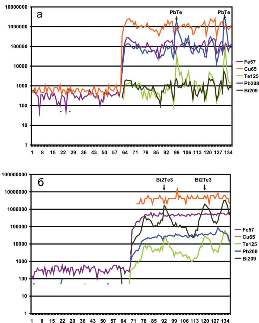
Рис. 4. Пример определения включения теллуровисмутита (а) и алтаита (б) в халькопирите черного палеокурильщика медно-цинково-колчеданного месторождения Яман-Касы (Maslennikov et al., 2009).
