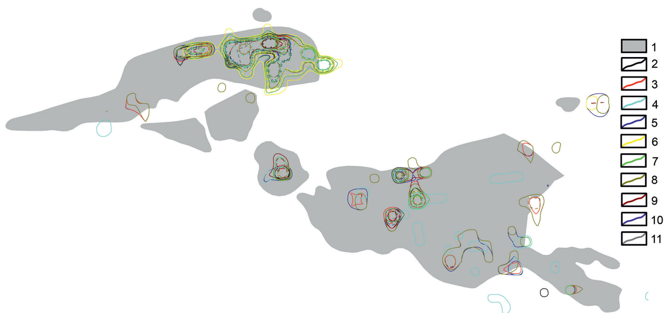
Рис. 7. Топоминералогическая карта Зирабулак-Зиаэтинского района.
