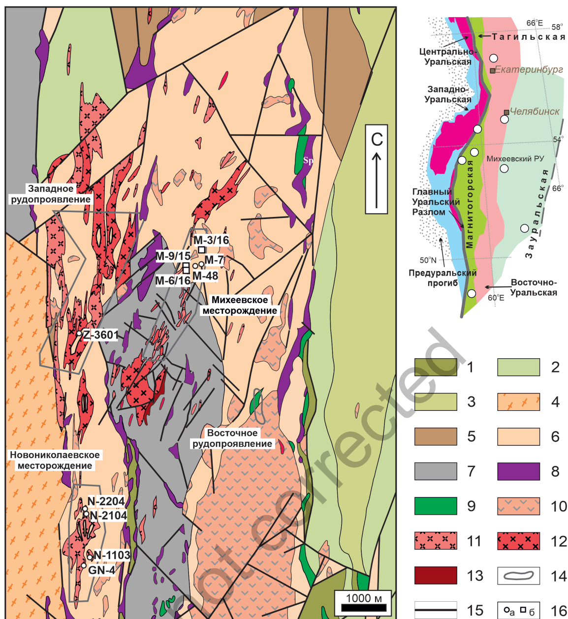
Рис. 1. Схематическая геологическая карта Михеевского рудного узла по данным ООО «Геосинтез» (Кузнецов и др., 2020) с упрощениями. На врезке показано положение Михеевского рудного узла на тектонической схеме Южного Урала по (Puchkov, 2017; Plotinskaya et al., 2017).
