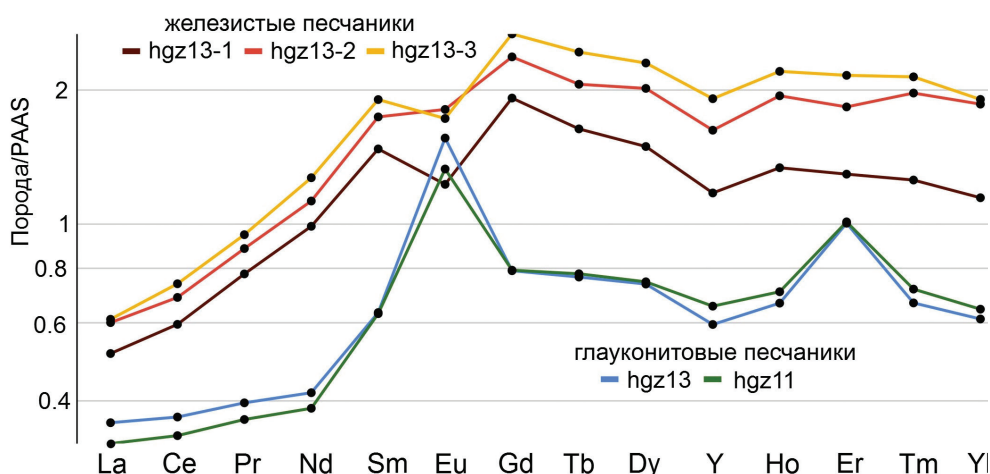
Рис. 9. PAAS-нормированные (Скляров и др., 2001) спектры РЗЭ для железистых и глауконитовых песчаников Агарцинского месторождения.
