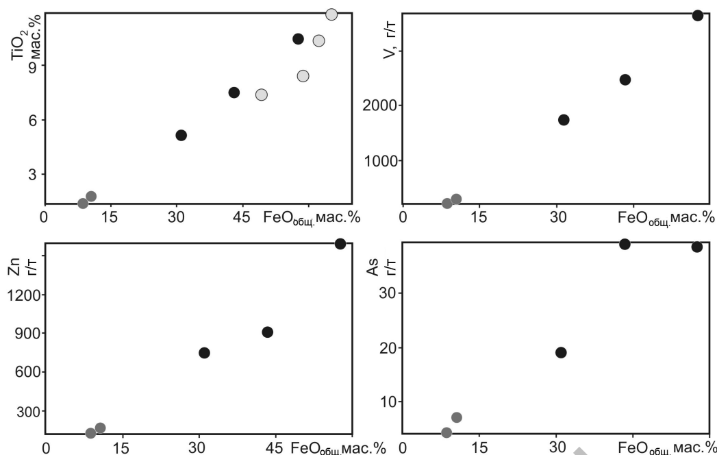
Рис. 11. Соотношение FeO общ. , TiO 2 , V, Zn и As в железистых песчаниках Агарцинского месторождения. Условные обозначения см. на рис. 7.
