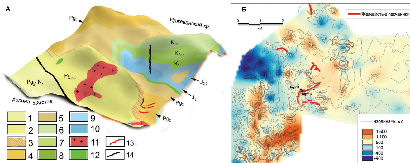
Рис. 2. Геологическая карта района на 3D поверхности рельефа (А) (Мкртчян, Туманян, 1963) и карта изодинам \Delta Z (Б) (Сепоян, 1956) с точками отбора проб hgз11 и hgз13.
